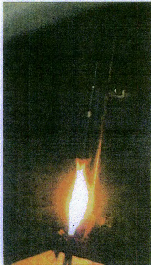
自己消火性の実証試験の例(UL垂直燃焼試験)
